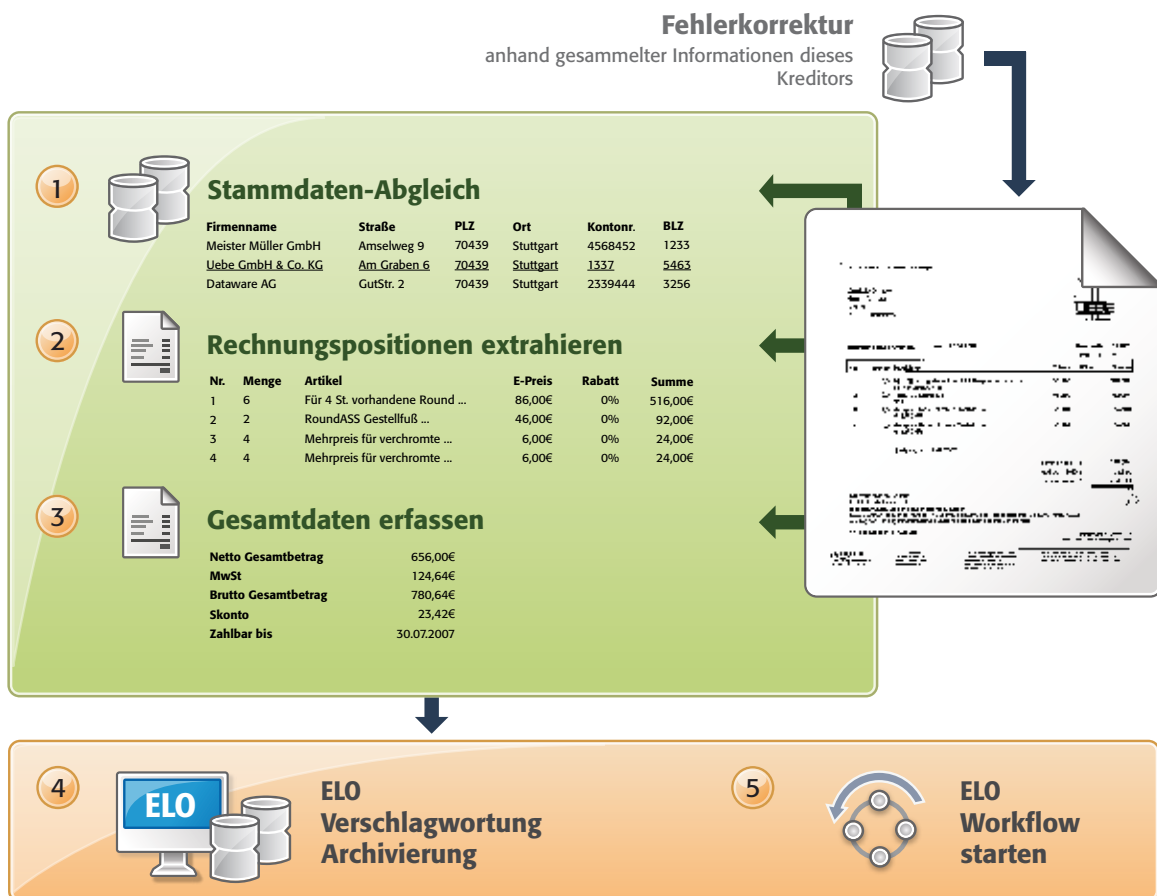
Abb. 3: Ausschnitt aus dem internen Ablauf des ELO DocExtractors
