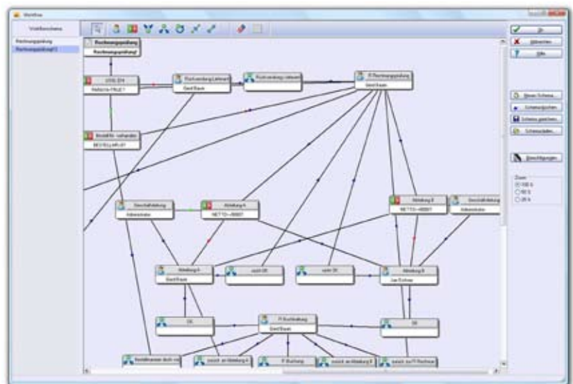
Abb. 2: Ausschnitt eines Freigabeworkflows in ELO
