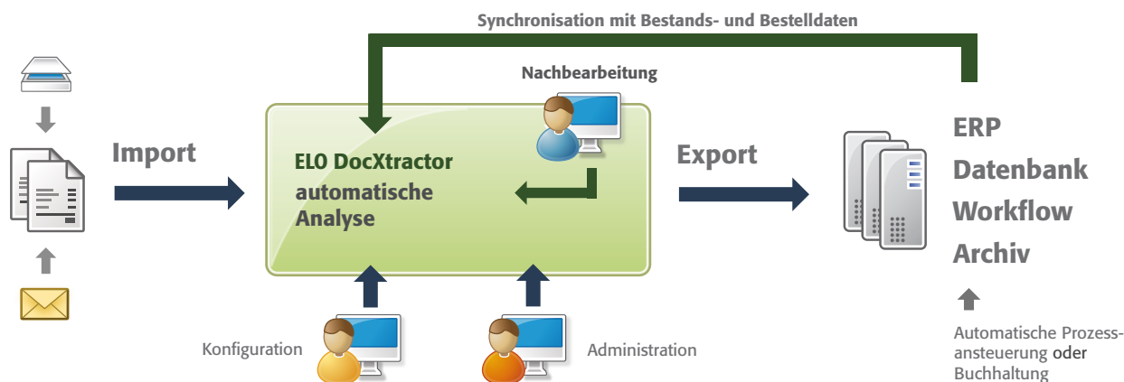
Abb. 1: Gesamtablauf des ELO DocXtractor
